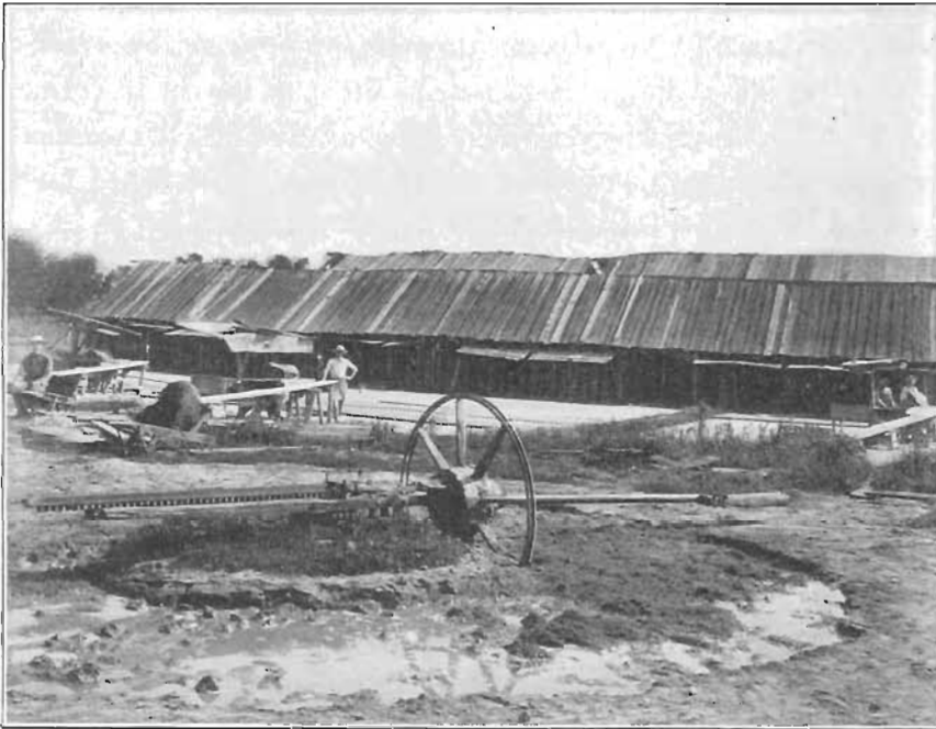
FIG. 16. Ring Pit, Carl Hagenmeister, Muscatine, Iowa.
