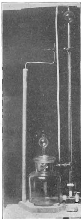
FIG. 2. The Seger Volumeter.
